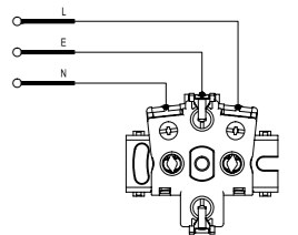
Schuko socket Πρίζα σούκο ασφαλείας
