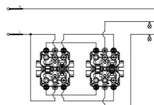
Double A/R switch Διακόπτης αλέρετουρ διπλός
