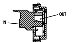
RJ45 DATA socket CAT6 Πρίζα RJ45 δεδομένων CAT6
