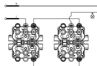
Double push button Μπουτόν διπλό
