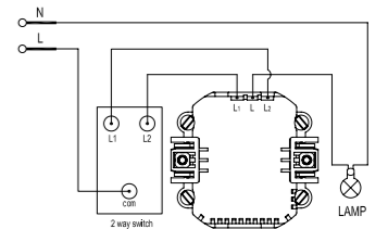
Dimmer for ordinary light Ρεοστάτης για απλό λαμπτήρα
