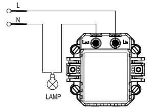
Dimmer A/R for LED light Ρεοστάτης A/R για λαμπτήρα LED
