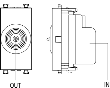
SAT socket Πρίζα δορυφορική τερματική
