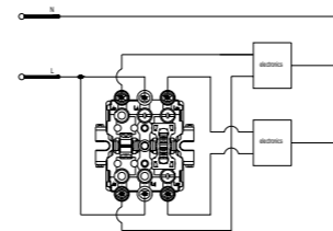
Double push button Μπουτόν διπλό
