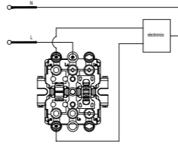
Push button Μπουτόν μονό
